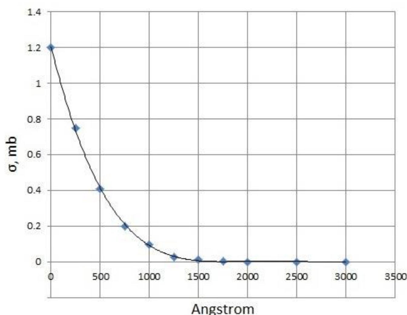
Зависимость сечения d+d реакции от глубины проникновения ионов дейтерия в алмазной мишени
