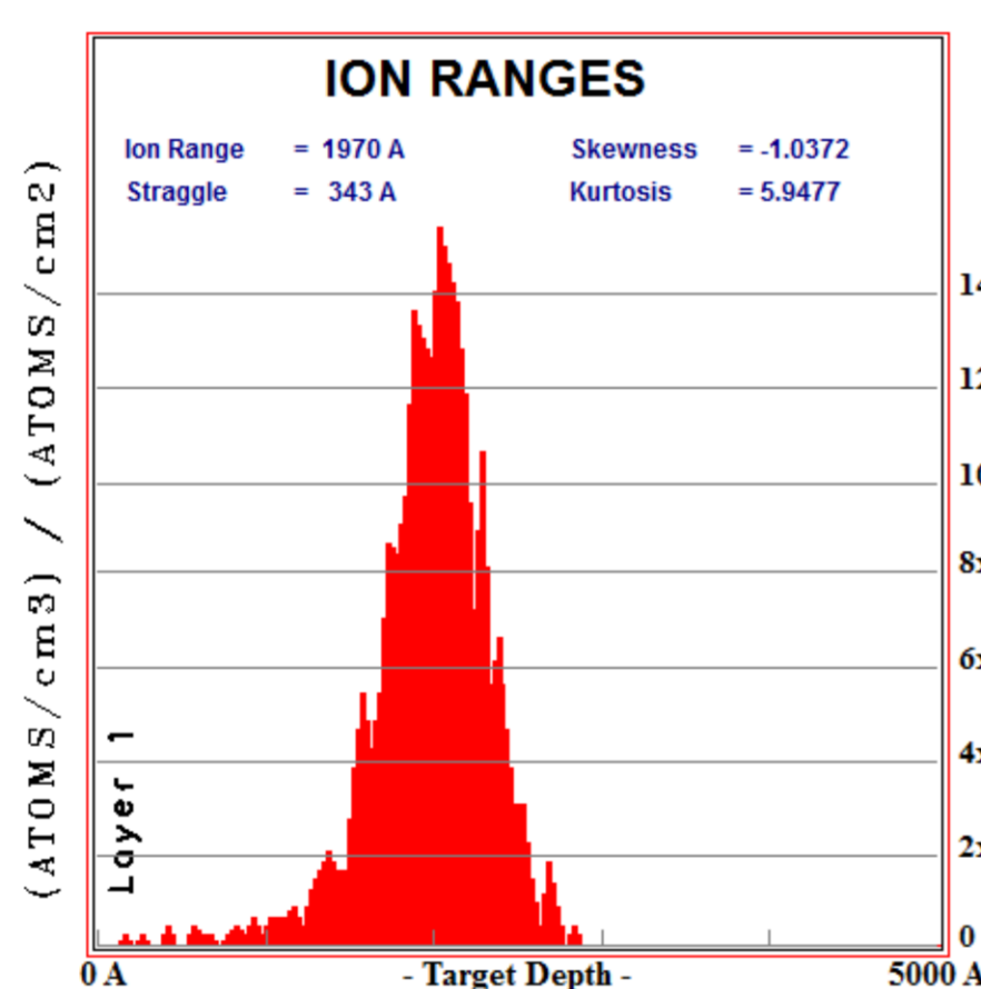
Распределение пробегов ионов дейтерия в алмазной мишени
