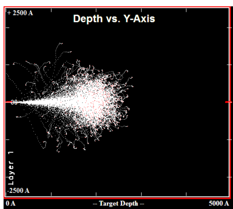
Моделирование прохождения ионов дейтерия в алмазной мишени
