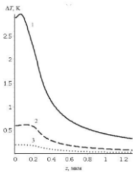
Рис. 1. Распределение температуры в Si по координате z . Расчёты проводились при x=0 , y=0 , при энергиях первичных электронов 5 (кривая 1), 10 (2), 15 (3) кэВ, токе зонда 10^{-7} А.
