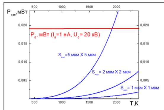
Рис. 3. Рассчитанные зависимости тепловой мощности, уносимой в вакуум излучением через площадки 5 \times 5 мкм и 1 \times 1 мкм от абсолютной температуры T этой площадки.
