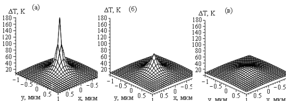
Рис. 2. Распределение температуры в Si (верхний рисунок), GaAs (средний рисунок) и CdTe (нижний рисунок) для энергии электронов зонда E_0=5 (а), 10 (б) и 20 (в) кэВ при токе зонда 10^{-7} А.
