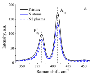
КРС спектры исходных и облученных пленок
