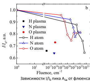
Зависимости I/I_0 пика A_{1g} от флюенса воздействующих частиц
