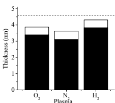
Толщины пленок \text{MoS}_2 без подложки на основании эллипсометрических данных
